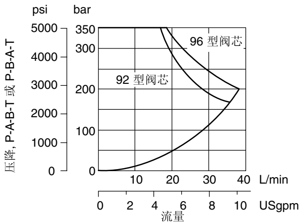
K(B)SDG4V-3-9*L-24 阀
