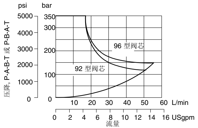
K(B)SDG4V-3-9*L-40 阀
