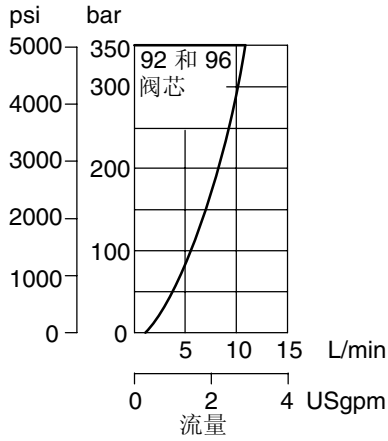
K(B)SDG4V-3-9*L-24 阀
