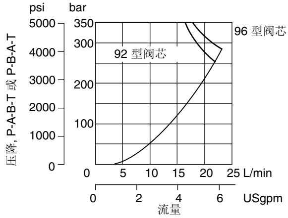
K(B)SDG4V-3-9*L-40 阀
